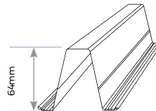
64 mm TOP HAT – 0.75 BMT: 64TH0.75 (1.26kg/m)
