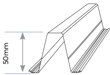
50 mm TOP HAT – 0.75 BMT: 50TH0.75 (1.09kg/m)
